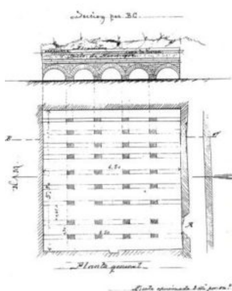
Figura 9. – Plano y alzado del praeurnium de la villa de las Torrecillas (Alcuéscar), En (Abascal, 1996: 277).
